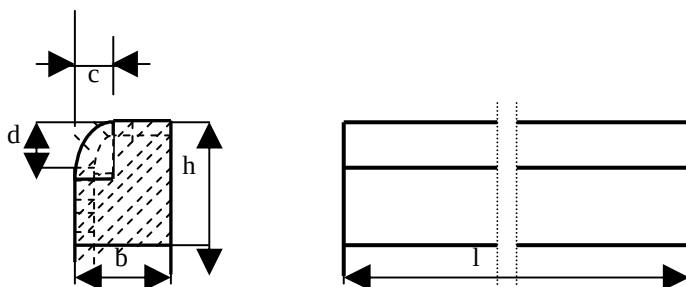
Rys. nr 1. Wymiarowanie krawężników.
