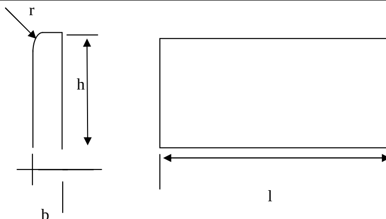
rysunek 1. Kształt betonowego obrzeża chodnikowego
